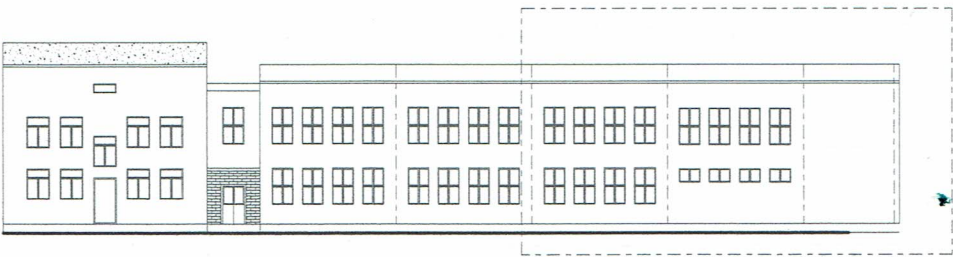
Budynek Szkoły - STEBANK gm. GRUNWALD Elewacja Frontowa: Północno-wschodnia
