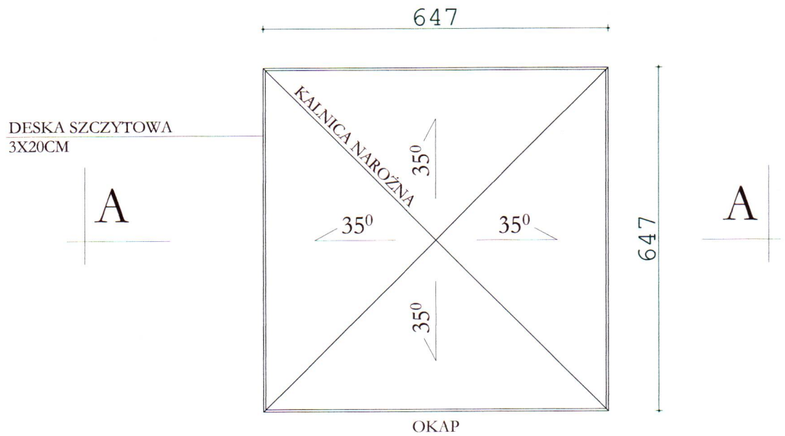
RZUT DACHU
