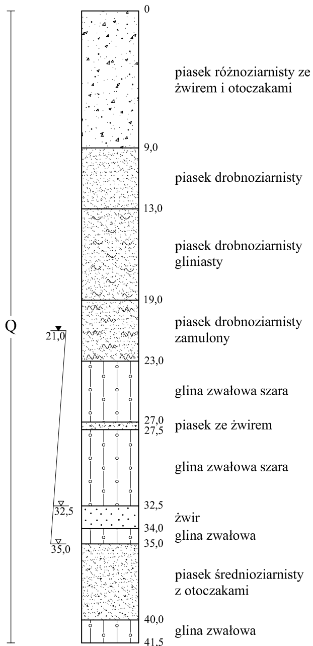
profil geologiczny
